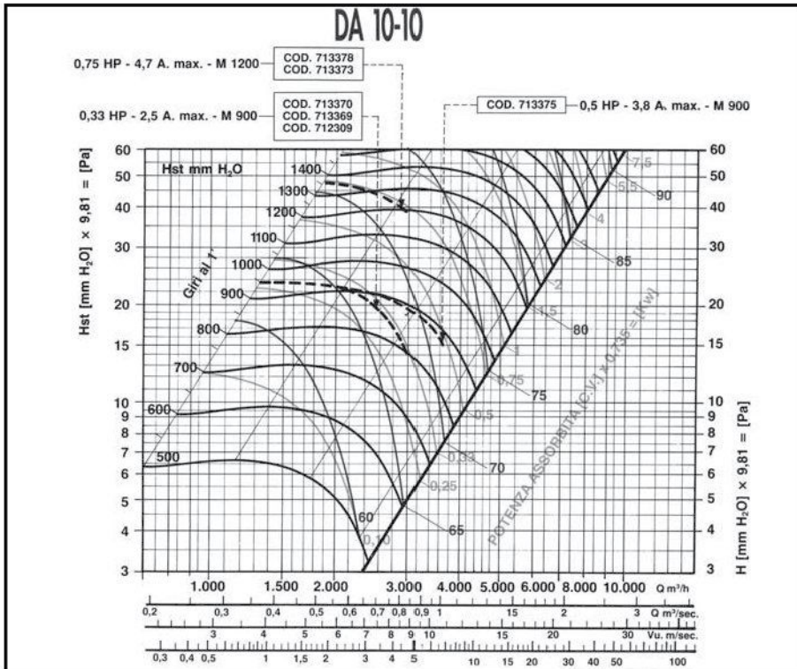
Καμπύλες ταχείας επιλογής ανεμιστήρων τύπου DA
