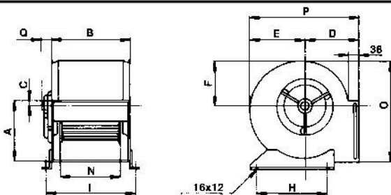
Διαστάσεις ανεμιστήρων (mm)
