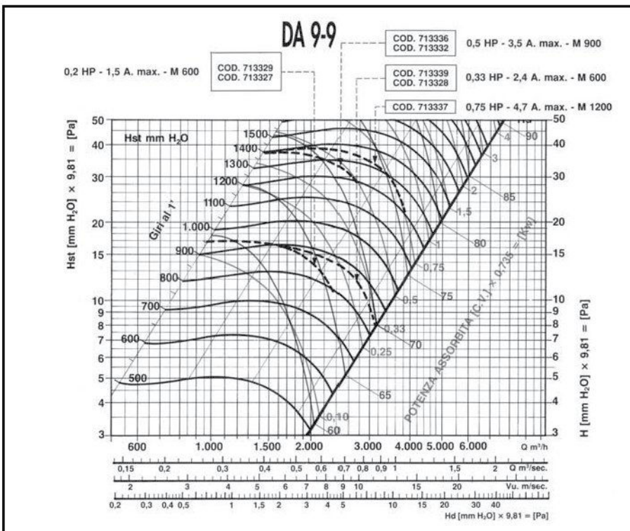
Διαγράμματα ταχείας επιλογής ανεμιστήρων τύπου DA
